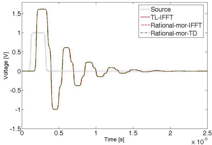
Fig. 1 – Tensione alla porta di uscita di una linea a vuoto.
