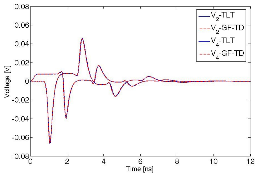
Fig.2 – Tensioni di near-end e far end in una linea dissipativa e dispersiva.
